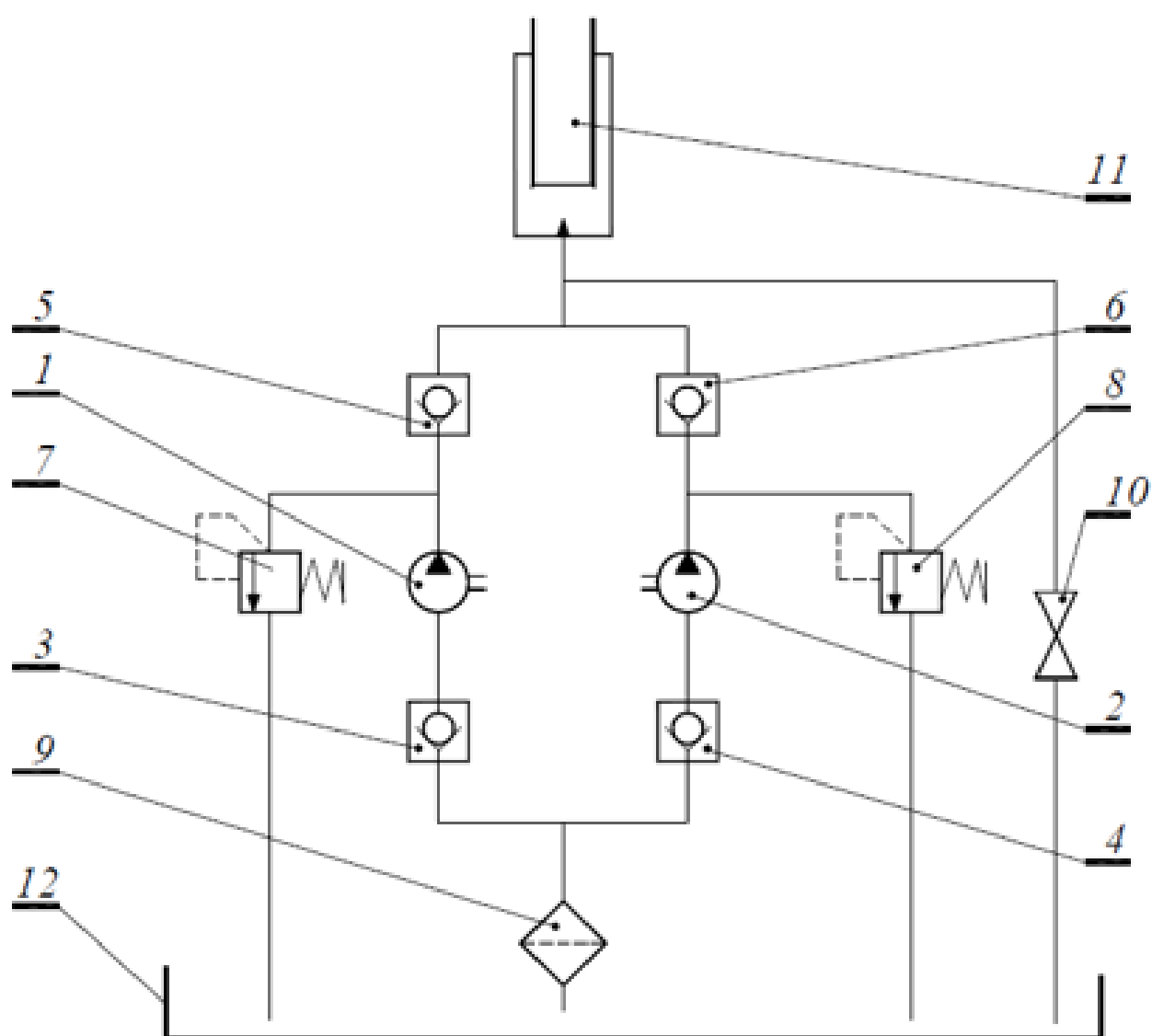
Schemat układu hydraulicznego
